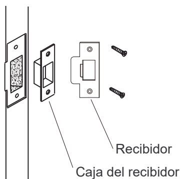
Figura 2: Instalación de cerraduras tubulares
