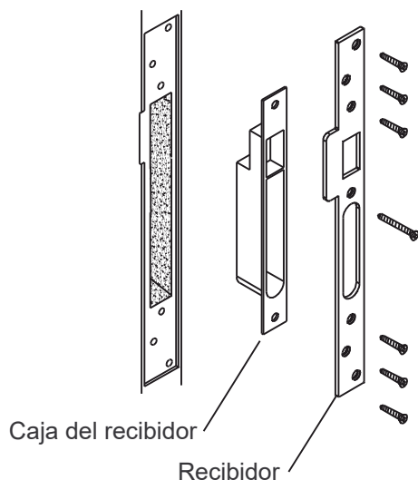
Figura 1: Instalación de cerraduras de embutir
